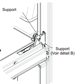
Détail A
